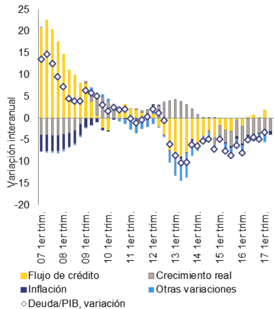
Gráfico 4.2.6: Desglose de las variaciones interanuales de los ratios deuda/PIB, datos trimestrales no consolidados, sociedades no financieras (SEC 2010), ES
